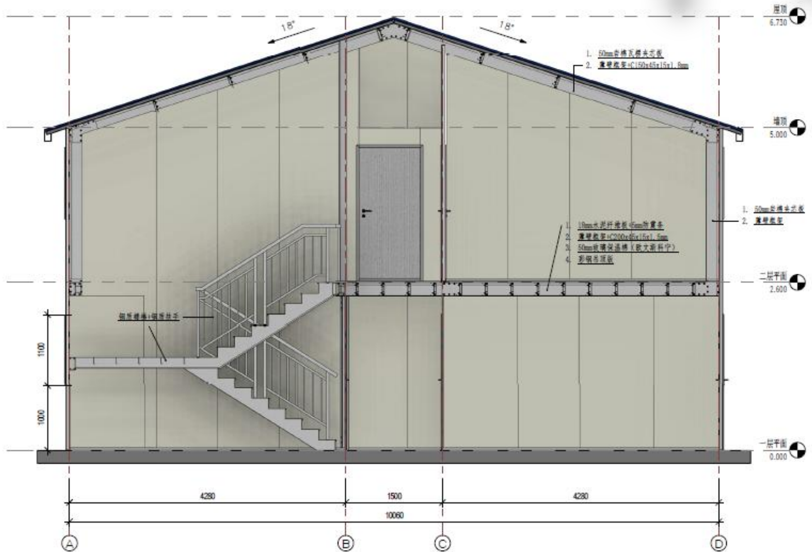
剖面图
