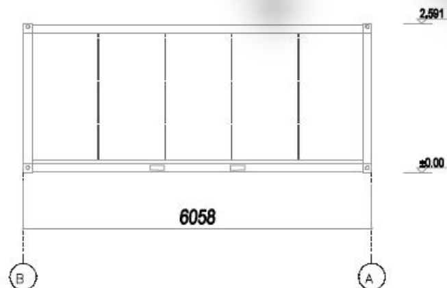
B~A轴立面图
