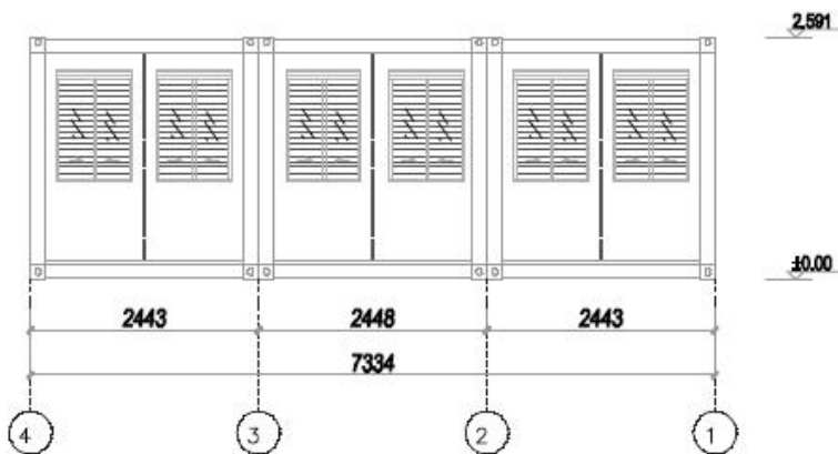
1~4轴立面图
