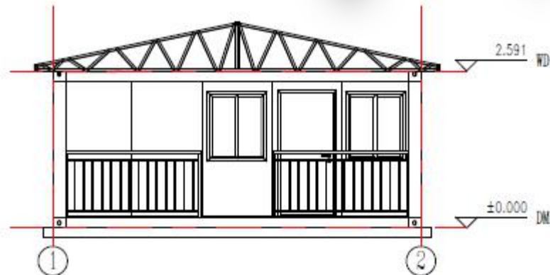
南立面图
