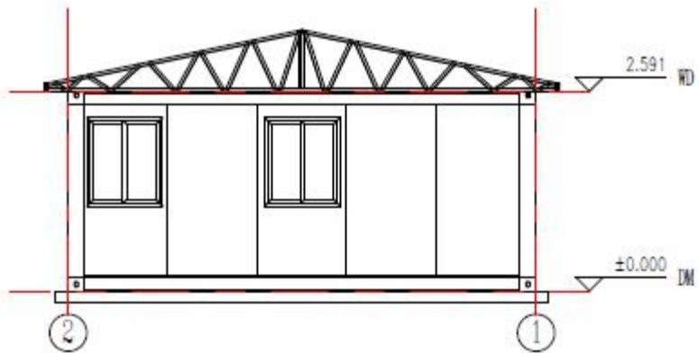
北立面图
