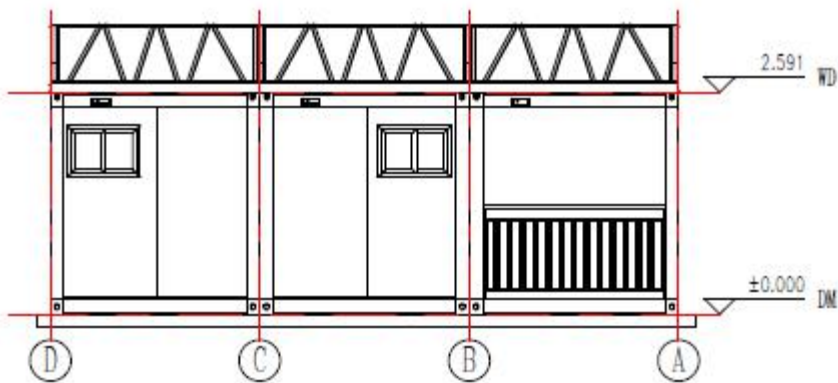
西立面图
