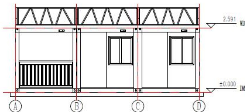
东立面图
